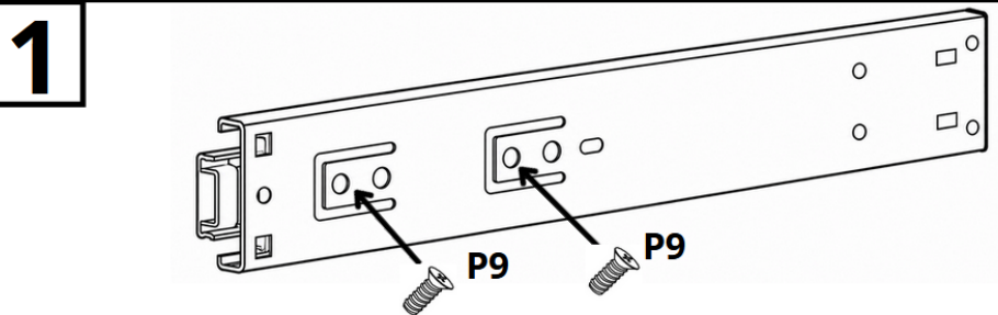
Widok tylnej części prowadnicy – poglądowy schemat rozmieszczenia okuć Rear view of the drawer slide – illustrative hardware placement diagram
